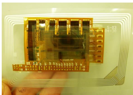
写真: 印刷できる商用 IC カード規格スピードの温度センサつき高速デジタル回路(左)と、温度センシング機能を搭載した電子タグの利用例(中、右)
