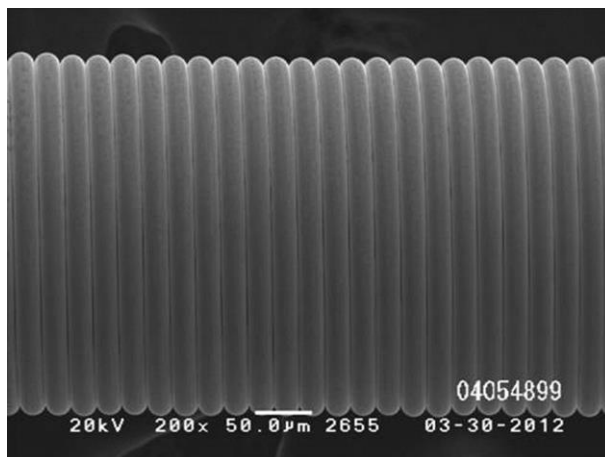
図 PtW8 極細線コイルリング材（線径 20\mu\text{m} 、コイル径 300\mu\text{m} ）
